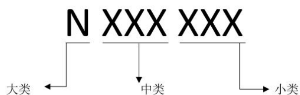
图 1 代码结构图
